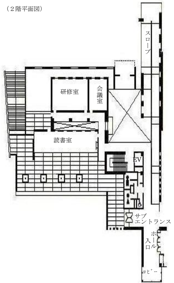
明石市立西部図書館平面図
