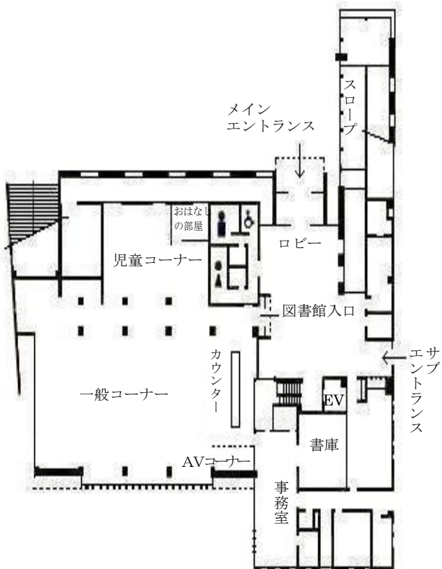
(1階平面図)
